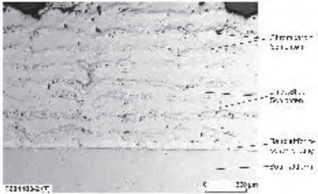
Bild 5: Schliffbild einer schichtweise aufgebauten Stahl-Cr 3 C 2 -Struktur
