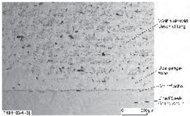
Bild 11: Schliiffbild einer Wolframkarbid-Beschichtung
