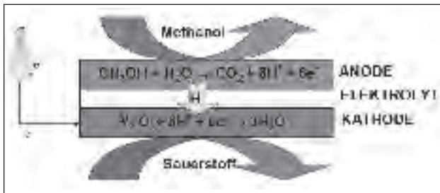
Abbildung 1: Schematische Darstellung der Abläufe in einer DMFC
