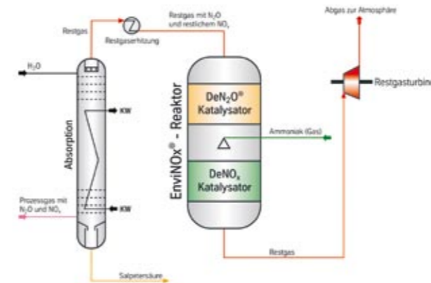
Abb. 2: Integration des EnviNOx®-Verfahrens in den Produktionsprozess
